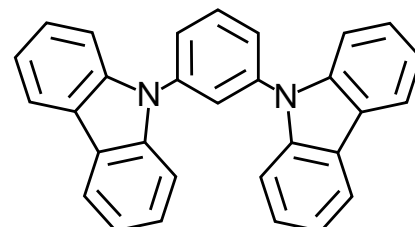
1,3-di-9-carbazolylbenzene
