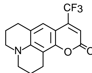
coumarin 153
