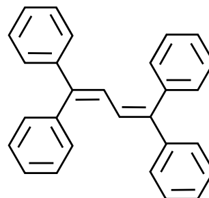
1,1,4,4-tetraphenyl-1,3-butadiene
